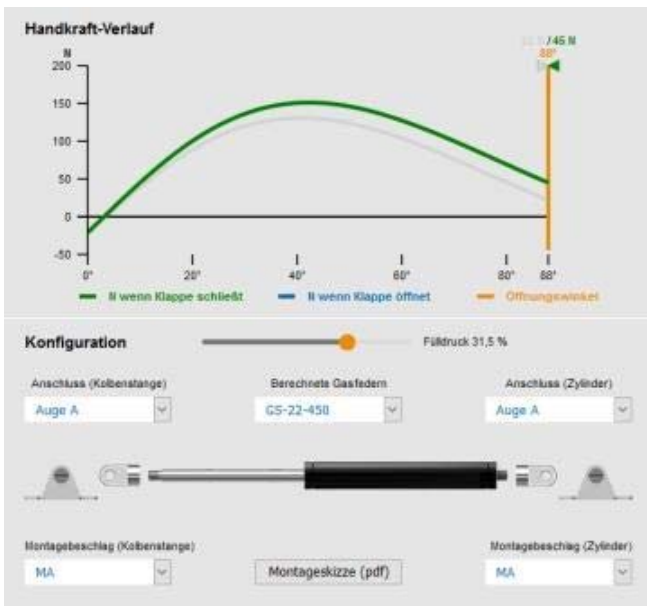
Bild 2 ACE Smart-Sizing Gasfeder Konfigurator-Graph 01.jpg
