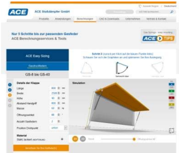
Bild 1 ACE Smart-Sizing Gasfeder Berechnung 01.jpg
