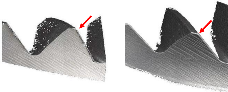
Schneidkante Gewindebohrer unbearbeitet (links) und bearbeitet (rechts) in OTEC-Maschinen
