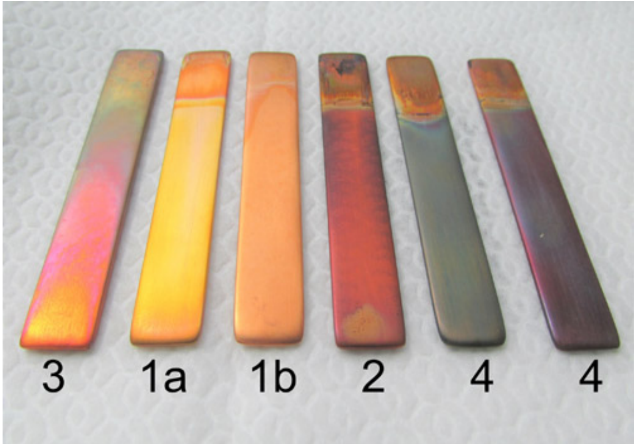
Bild Nr. 19-01 OE_Kupfertest.jpg. Verschiedene Korrosionsgrade vom Kupferstreifentest nach ASTM D 130 - Produkte von Oemeta bei 1a (2. v li).
