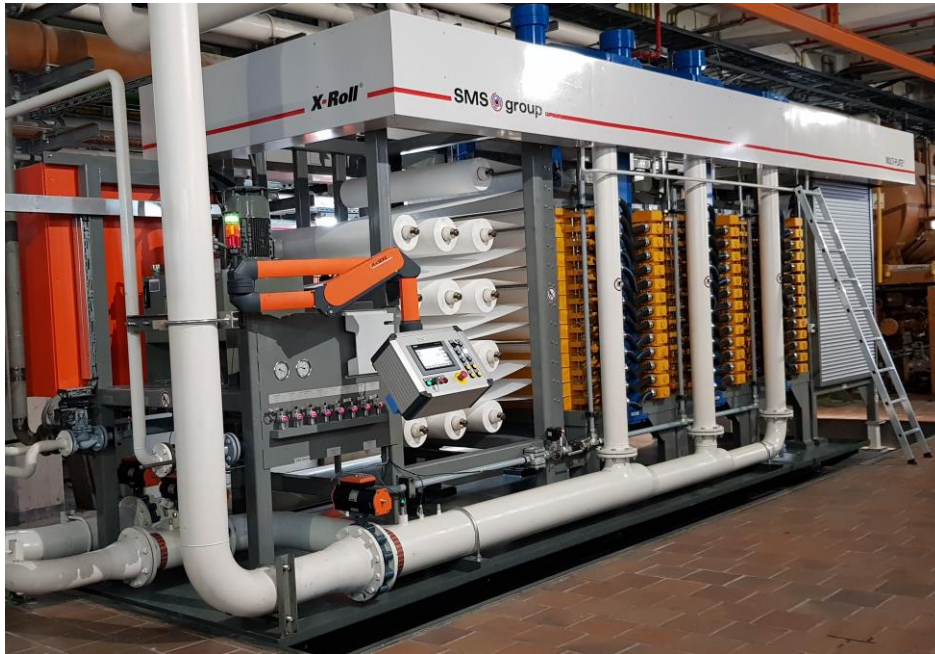
Multi-Plate®-Filter in der Endmontage bei Hydro.
