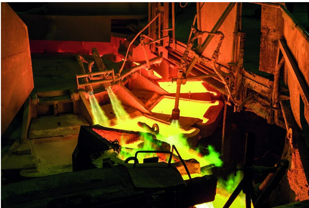
Anodengießrad.
