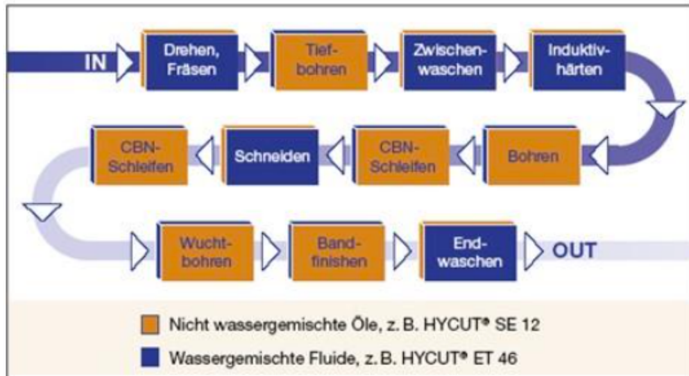
Bild 6: Blocklayout der Kurbelwellen-Fertigungslinie
